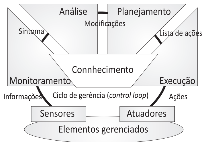
Figura 2.2. Ciclo de gerência ( control loop ) – Adaptado de [2].
