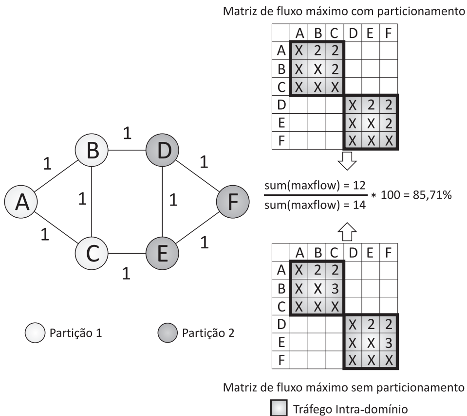
Figura 3.13. Cálculo da manutenção do somatório do fluxo máximo
