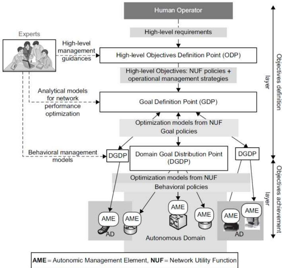
Figura 2.7. Visão global do ANEMA [8].
