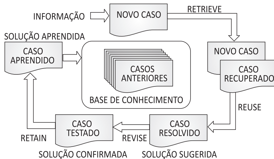
Figura 3.15. O ciclo do algoritmo 4R – Adaptado de [9]
