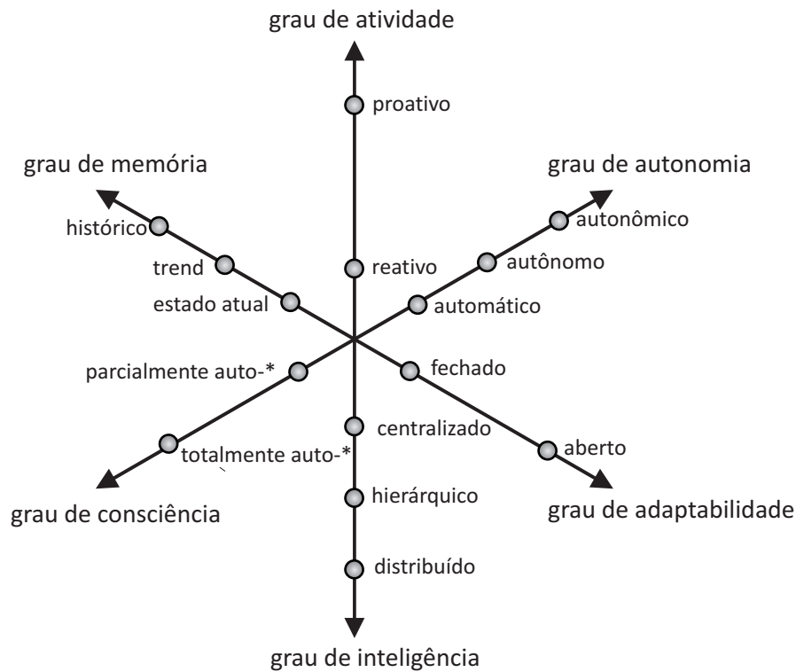
Figura 2.4. Classificação dos sistemas autônomicos [4].
