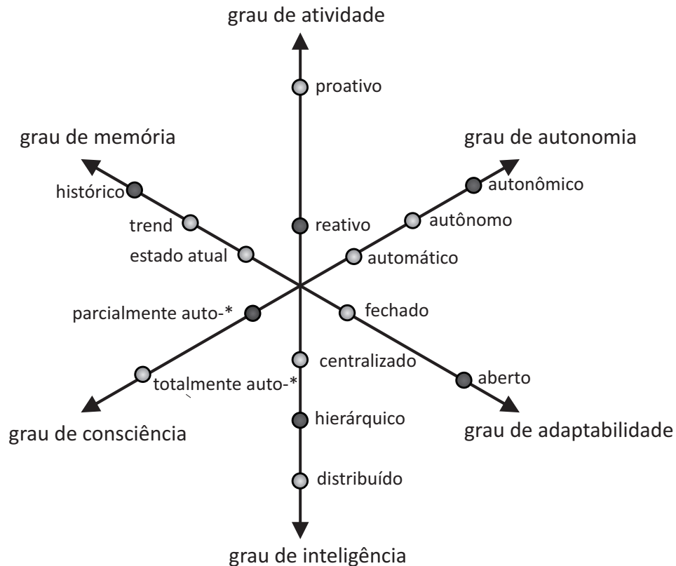
Figura 4.7. Classificação do arcabouço proposto segundo [4].
