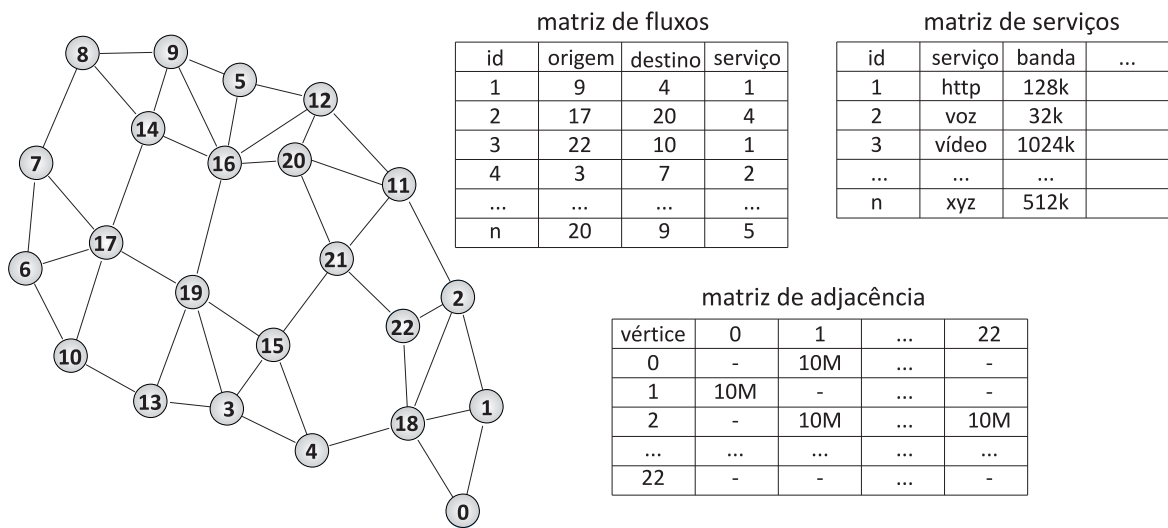
Figura 3.8. Exemplo ilustrativo da entrada do arcabouço autônomo
