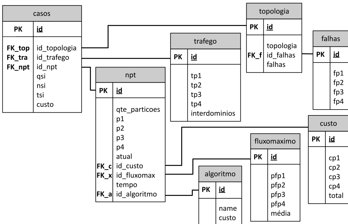
Figura 3.16. Modelo de dados para tomada de decisões
